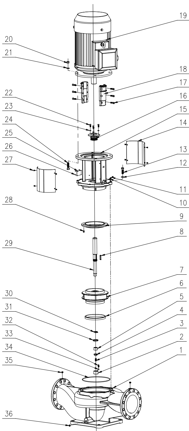
DP200~300分解图
