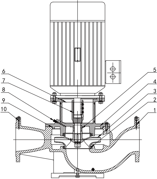
结构图 ( DP32~DP150 )
