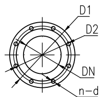
进出口法兰尺寸
